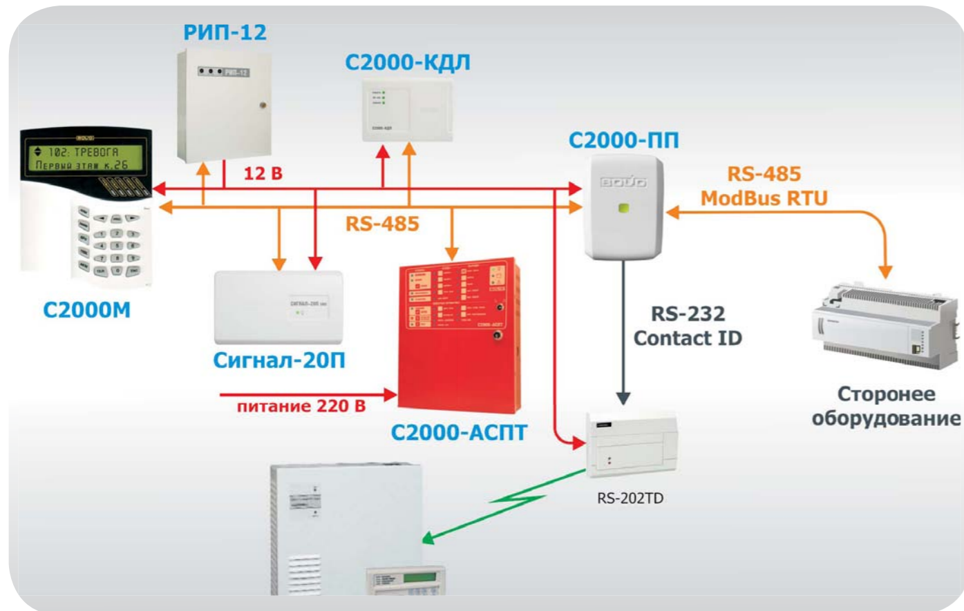
Рисунок 54. Применение «С2000-ПП» в ведомом режиме
