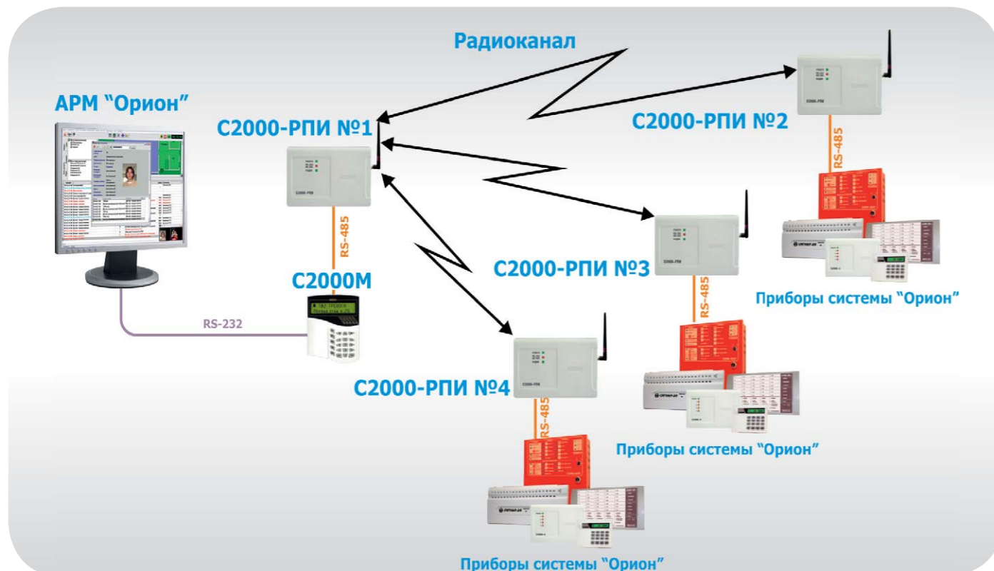
Рисунок 75. Структурная схема использования «С2000-РПИ» с АРМ «Орион» и «С2000М», соединение «точка-многоточие»
