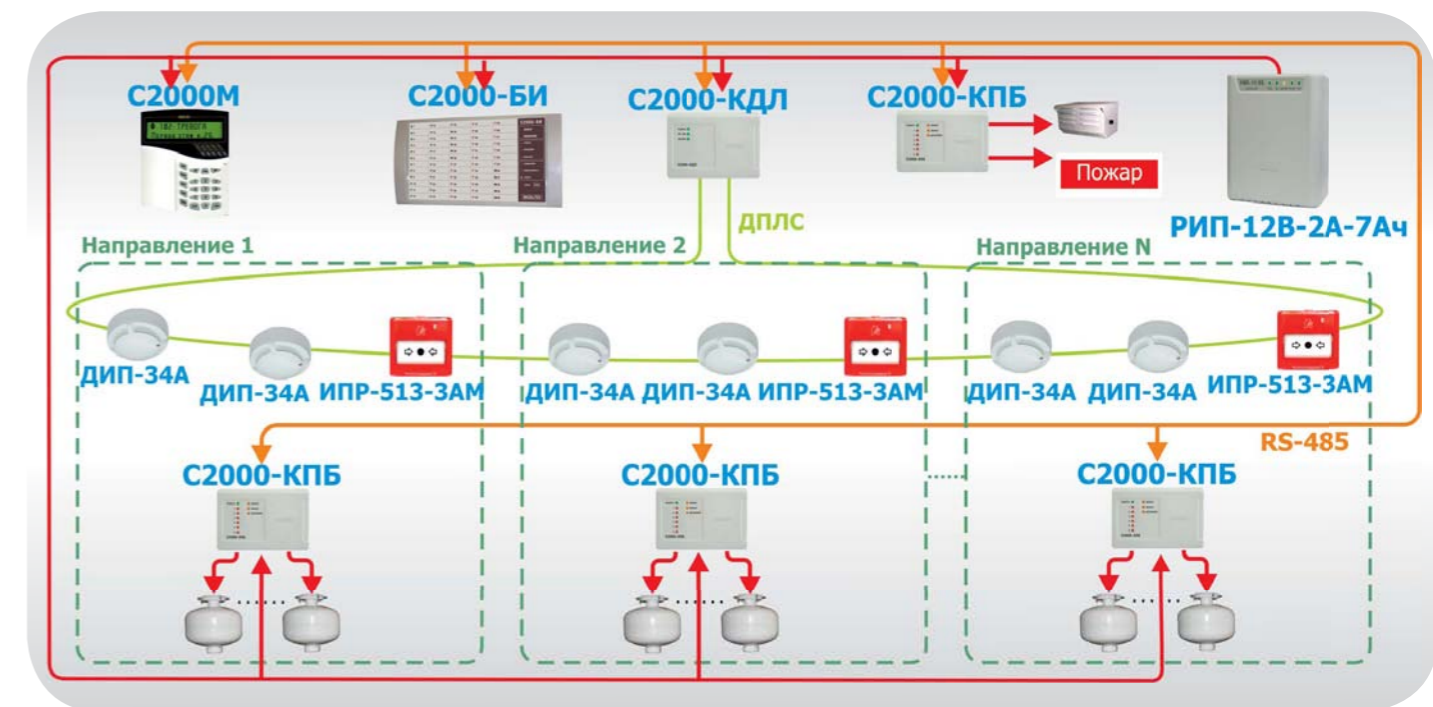
Рисунок 26. Система тушения с использованием приборов «С2000-КДЛ» и «С2000-КПБ»
