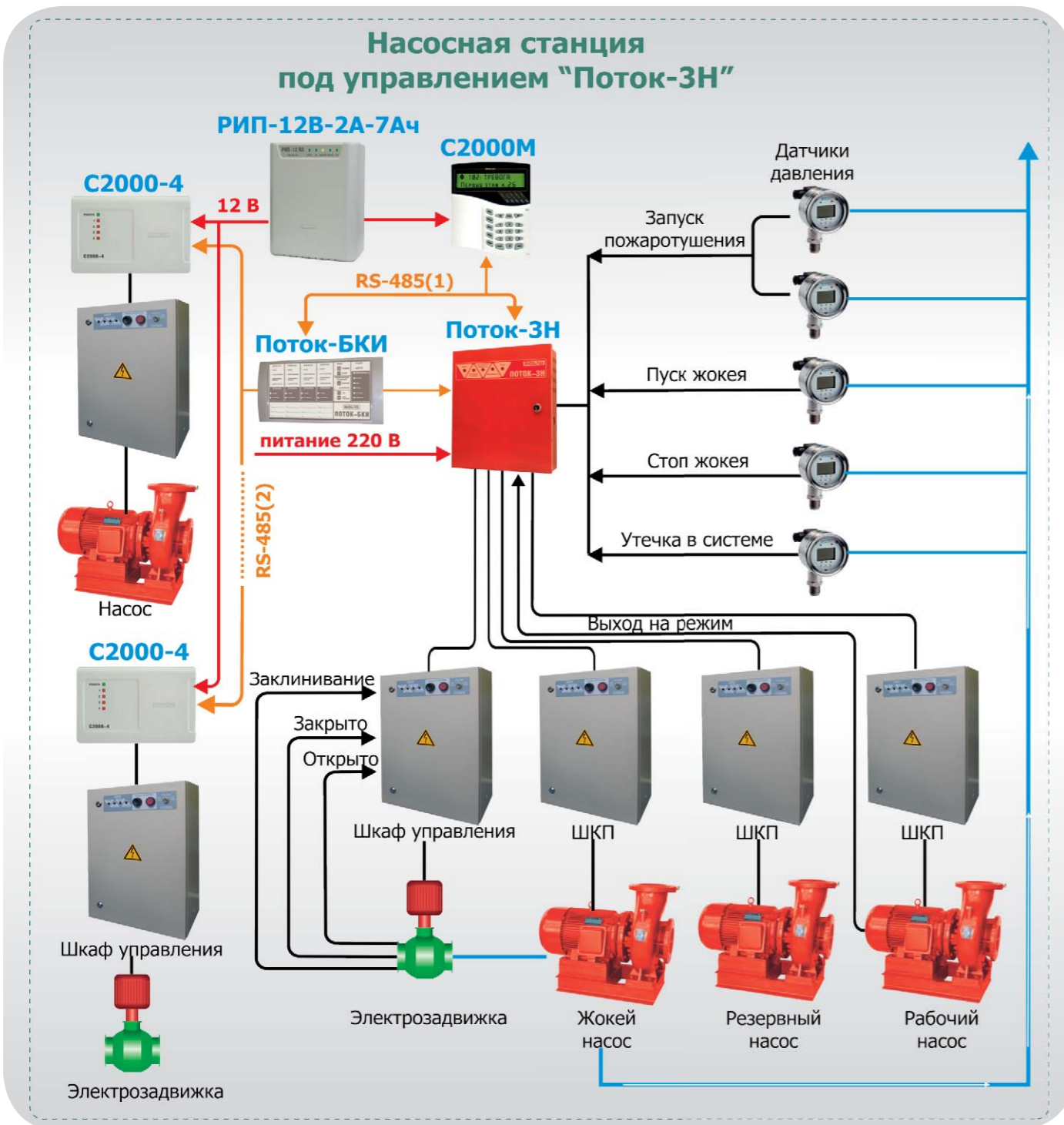
Рисунок 21. Система водяного пожаротушения
