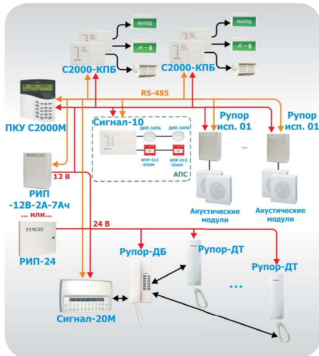
Рисунок 17. Пример СОУЭ 4-го типа с автономным комплексом обратной связи
