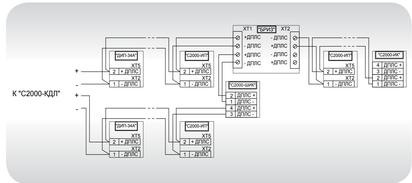
Рисунок 84. Схема подключения адресных извещателей в ДПЛС с топологией построения «кольцо»
