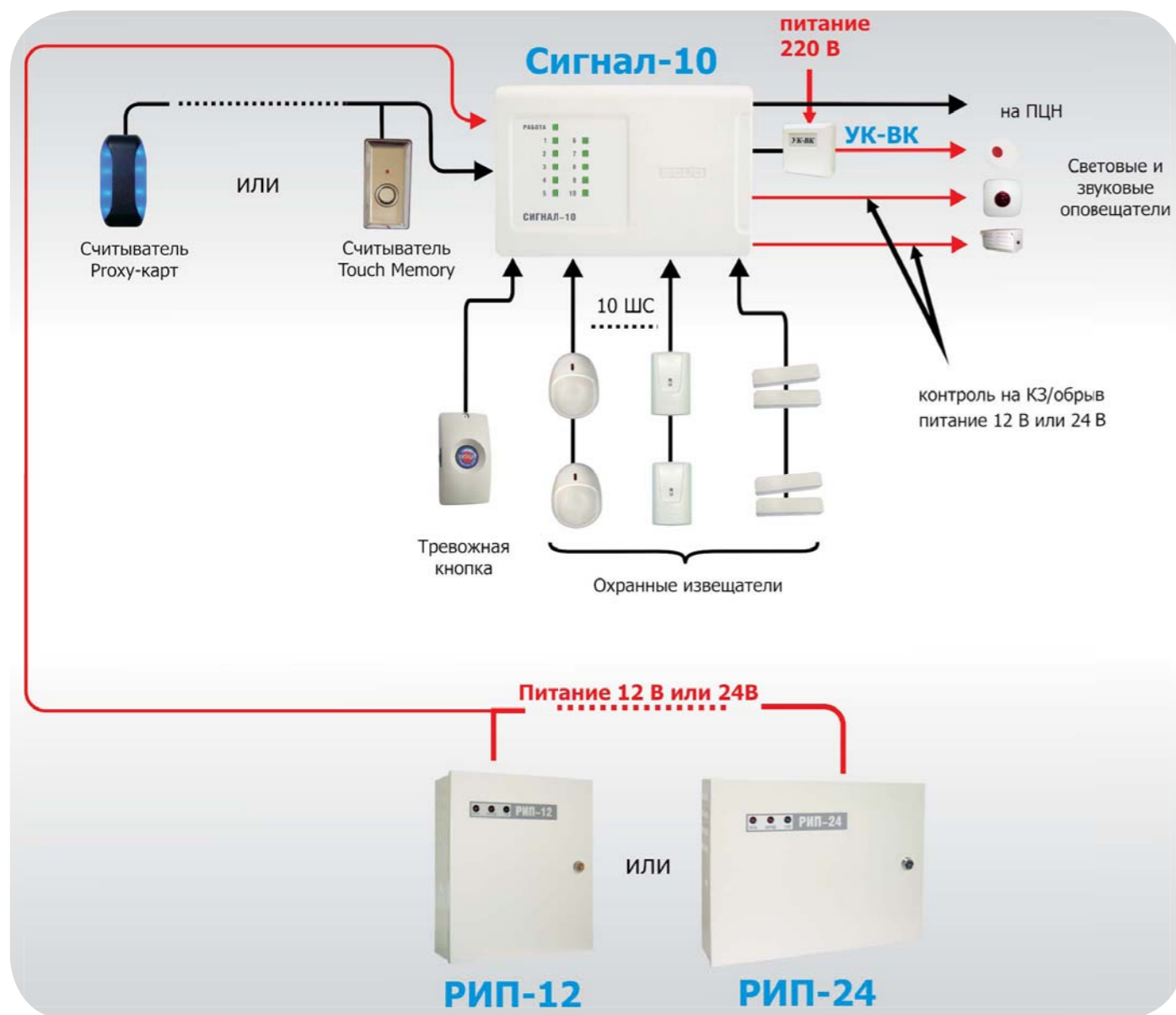
Рисунок 29. Автономное использование прибора «Сигнал-10»
