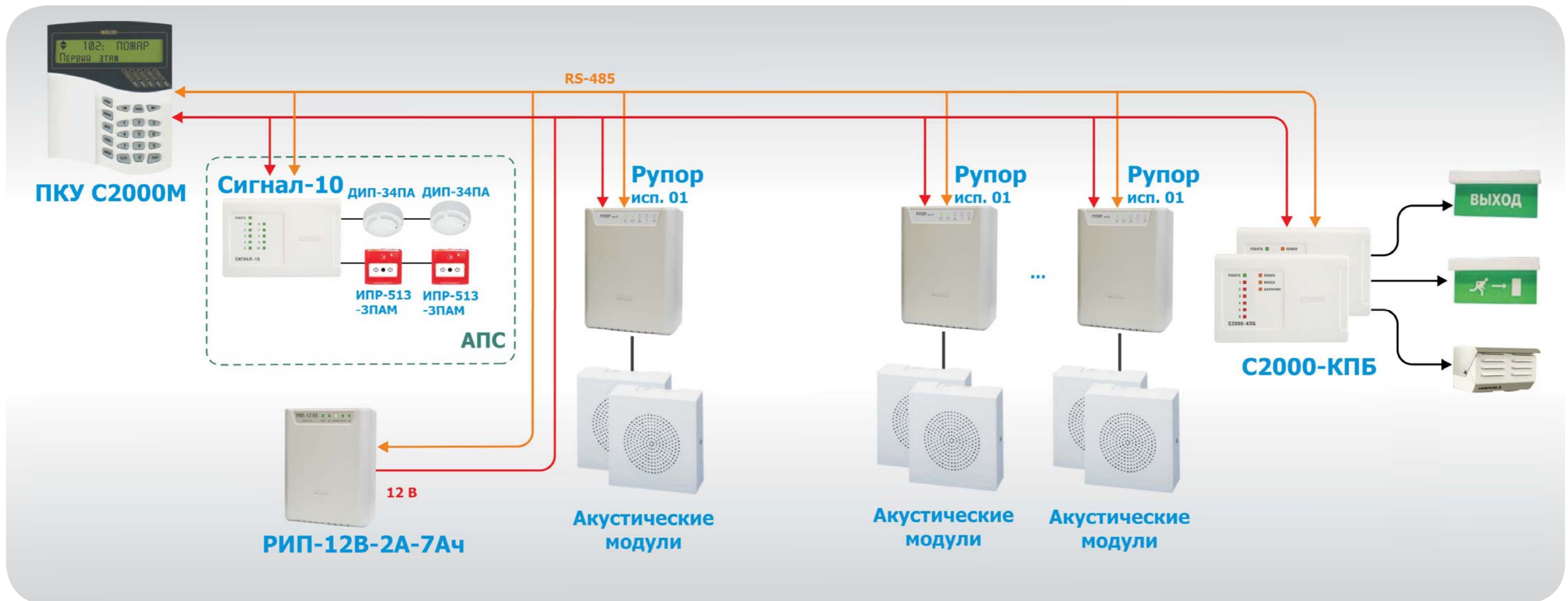
Рисунок 16. Пример СОУЭ 3-го типа с несколькими зонами оповещения
