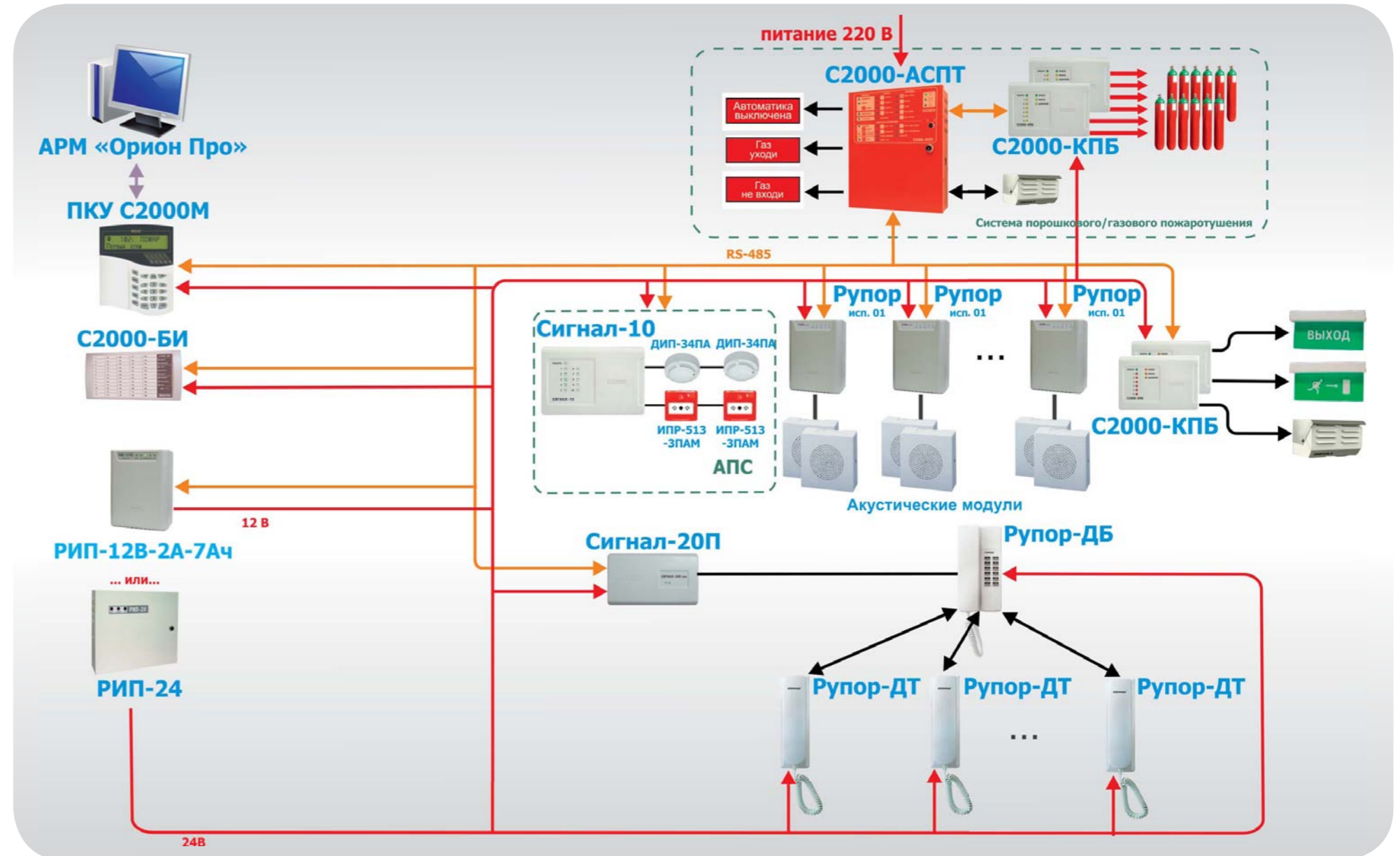
Рисунок 18. СОУЭ 5-го типа с комплексом обратной связи, входящим в состав ИСО «Орион»
