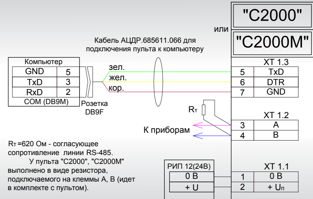
Рисунок 58. Схема подключения пульта «С2000»/ «С2000М» к персональному компьютеру с АРМ «Орион Про»
