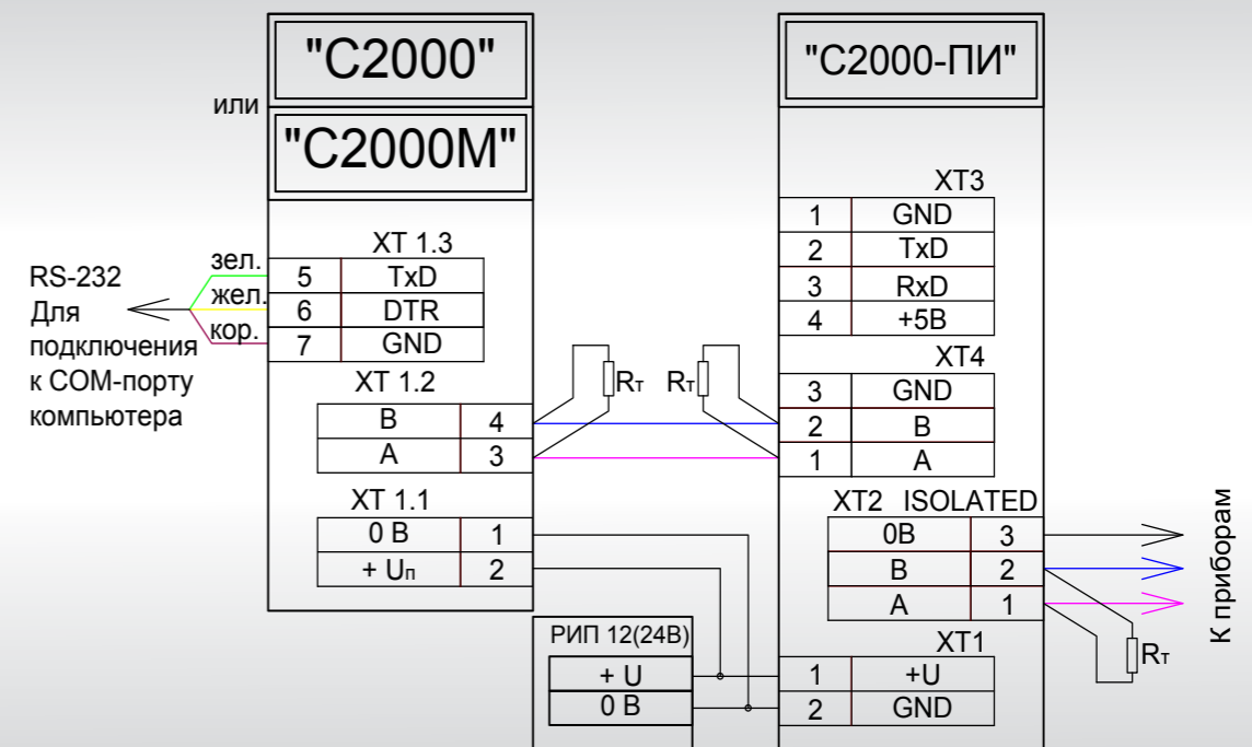
Рисунок 59. Схема подключения пультов «С2000»/ «С2000М» к персональному компьютеру с АРМ «Орион Про» с гальванической изоляцией интерфейса RS-485
