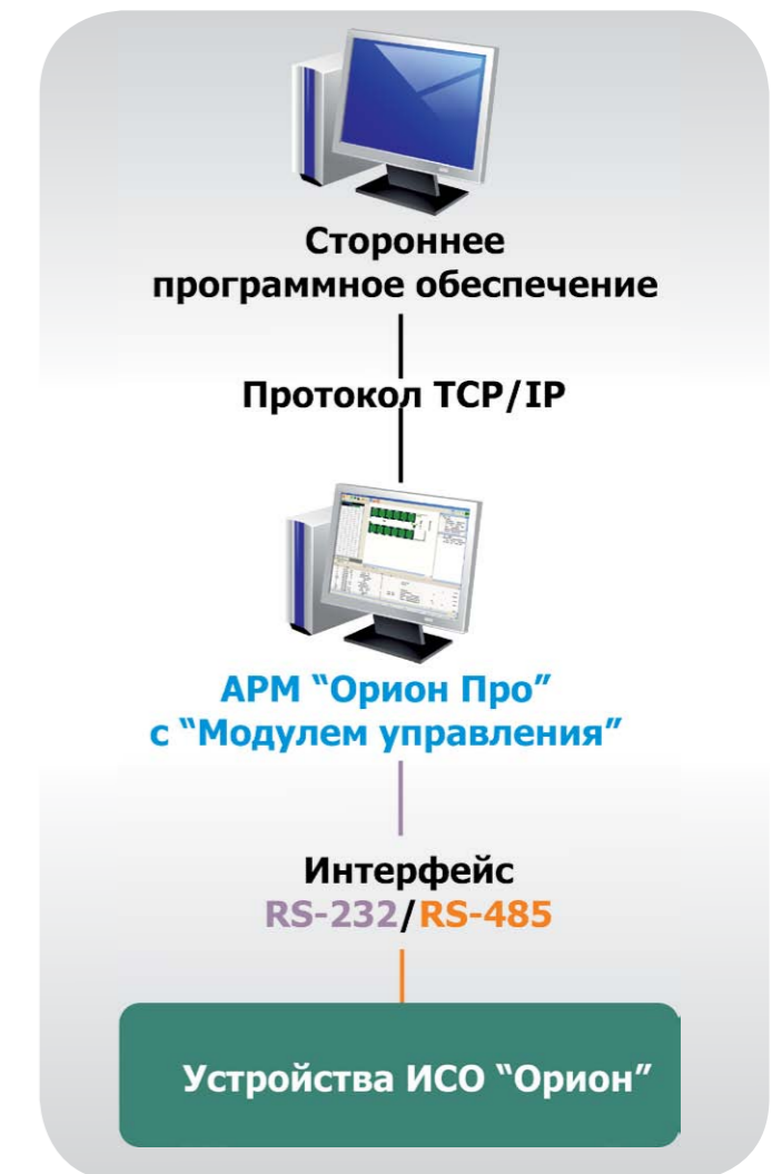
Рисунок 56. Интеграция с устройствами посредством интерфейса «Модуля управления» в АРМ «Орион Про»
