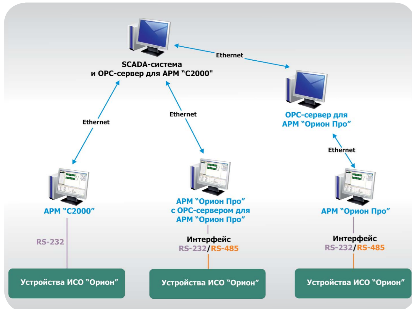
Рисунок 57. Передача данных в SCADA-системы
