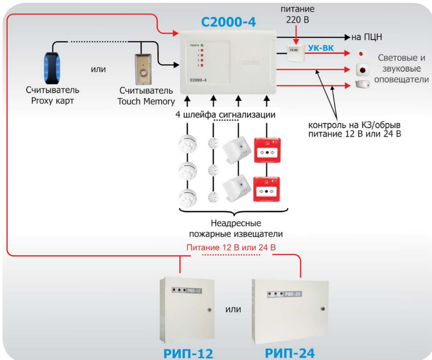
Рисунок 4. Использование прибора «С2000-4» в автономном режиме
