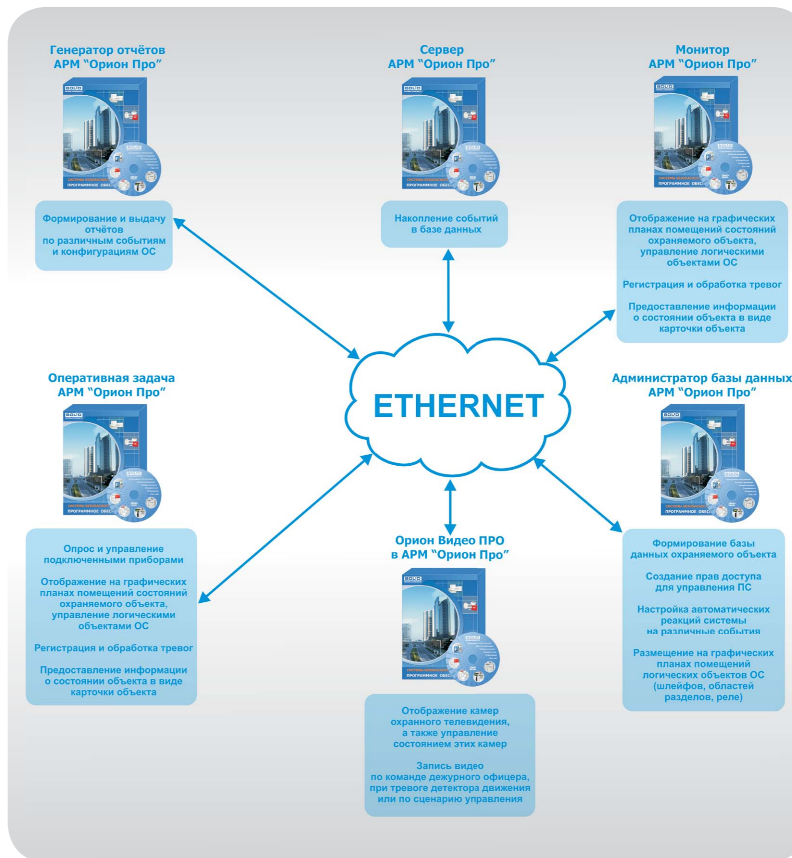
Рисунок 35. Функционал модулей программного обеспечения
