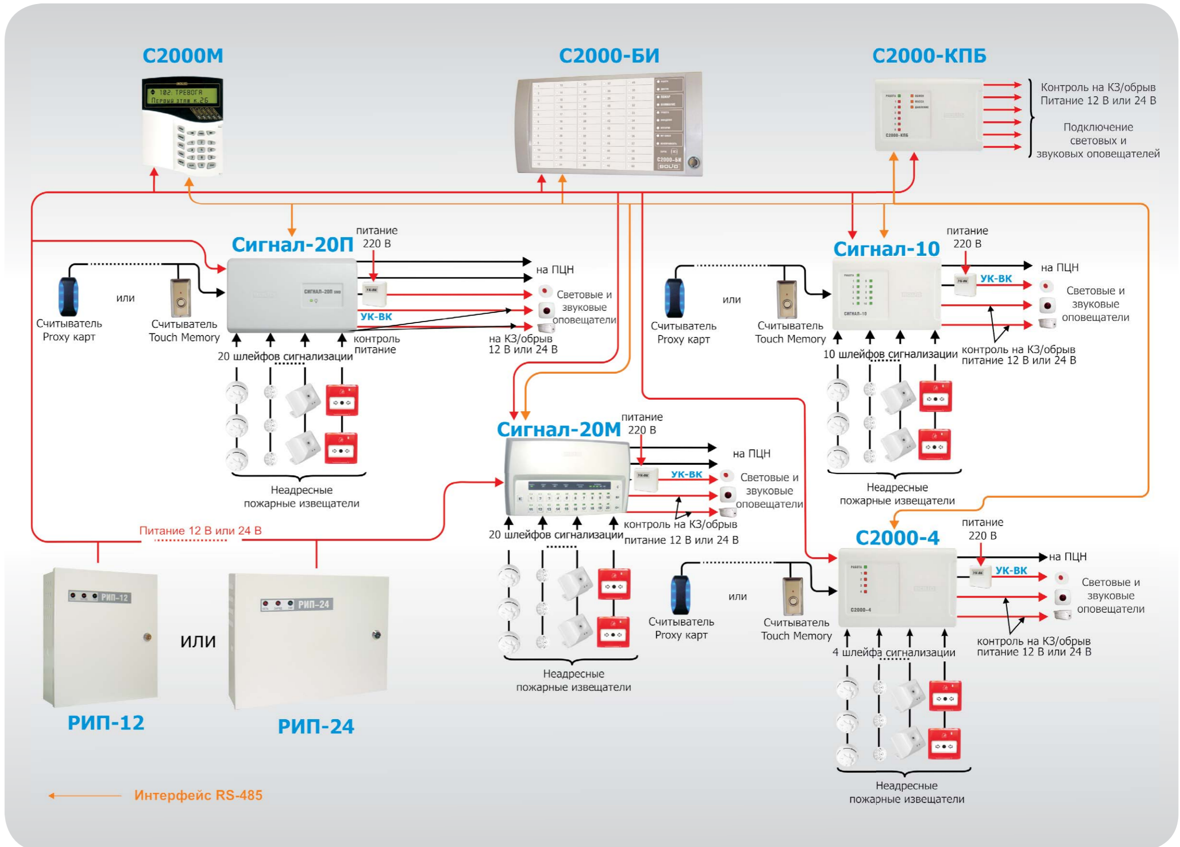
Рисунок 7. Неадресная система пожарной сигнализации в ИСО «Орион»
