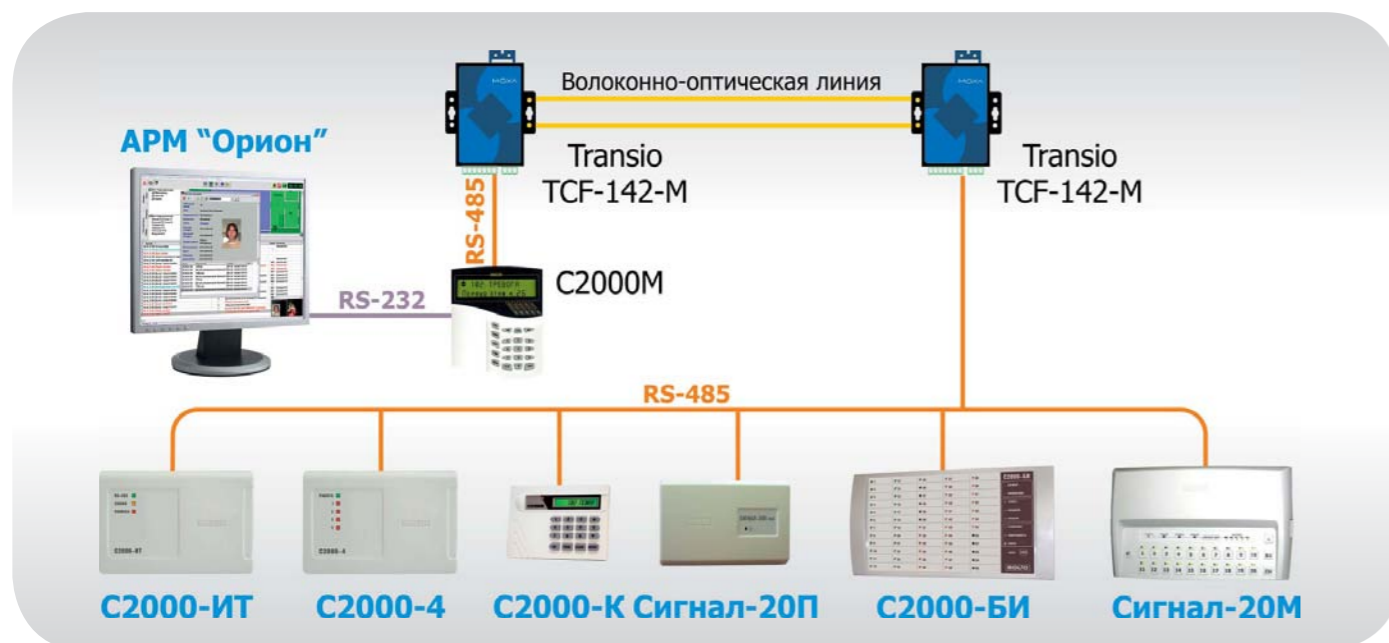
Рисунок 73. Структурная схема использования Transio TCF-142-M с АРМ «Орион» и «С2000М»
