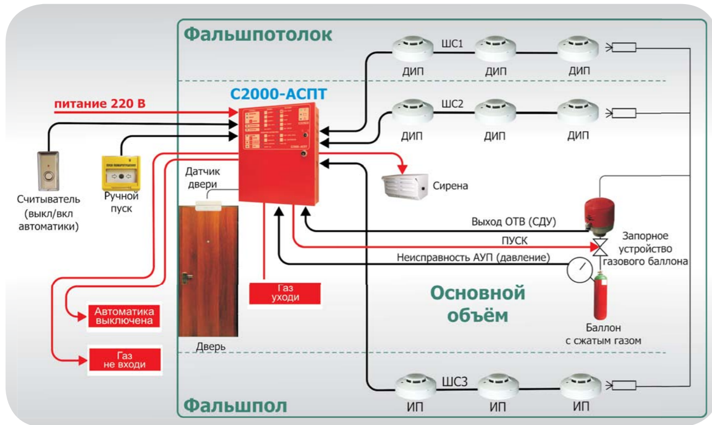
Рисунок 19. Автономная установка газового пожаротушения
