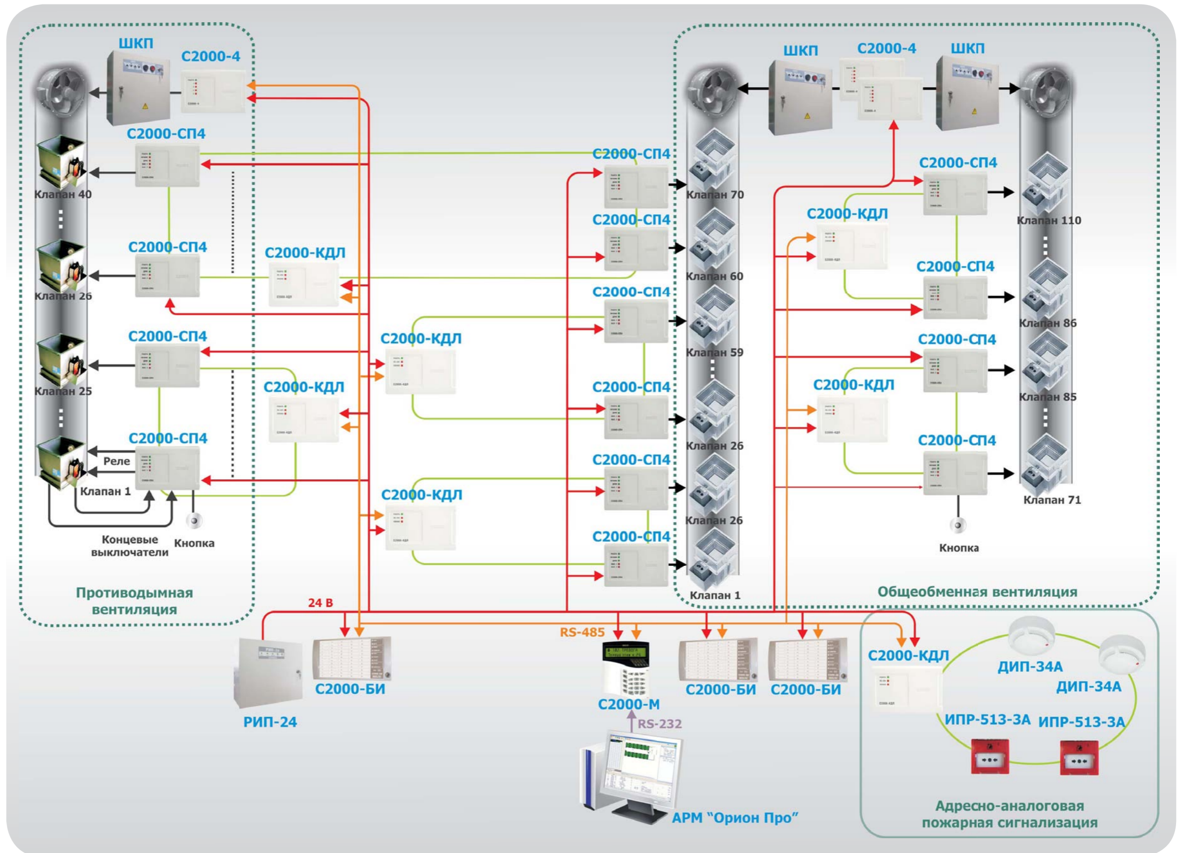
Рисунок 27. Структурная схема управления противопожарными клапанами
