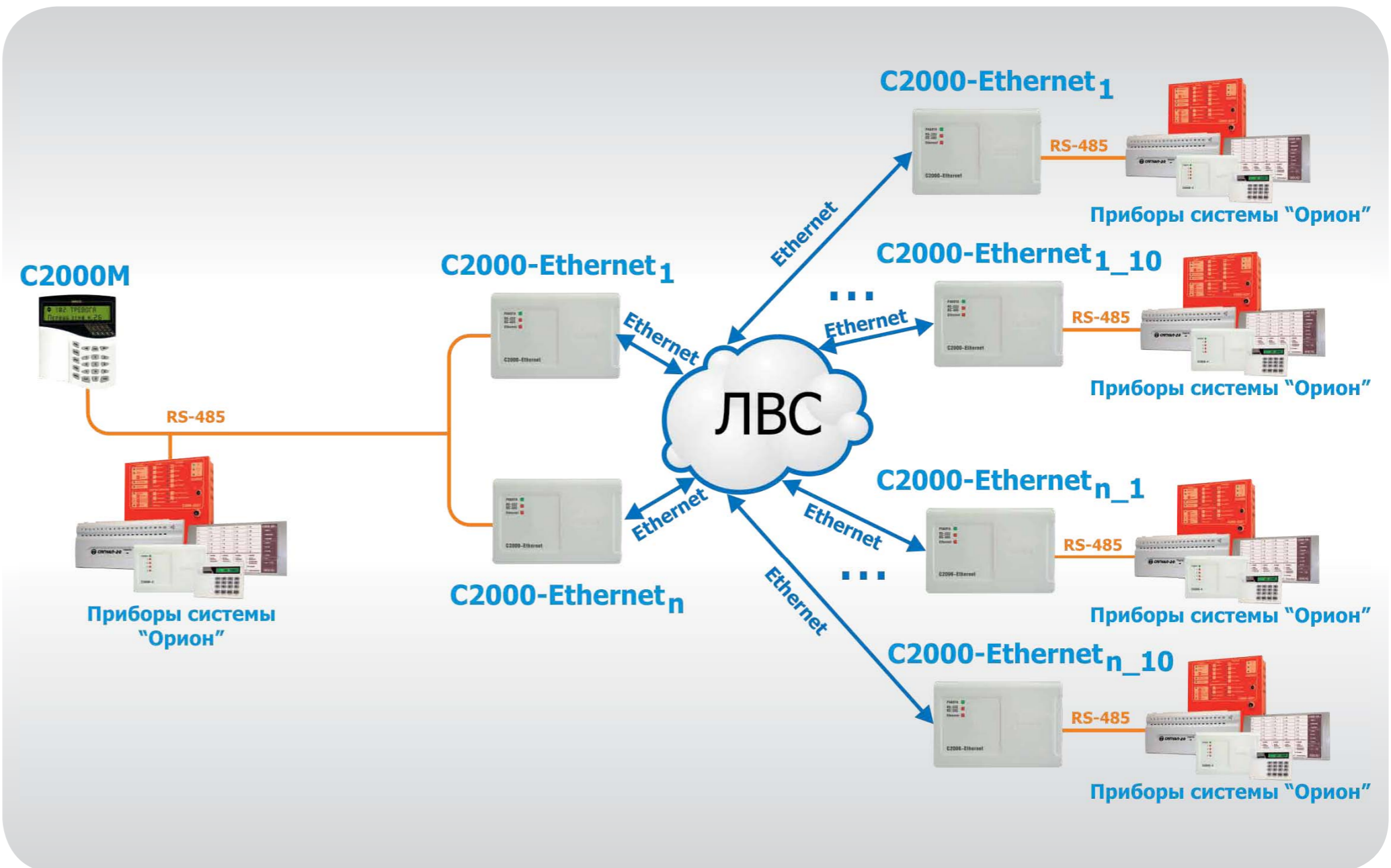
Рисунок 72. Структурная схема использования «С2000-Ethernet» с АРМ «Орион» и «С2000М»
