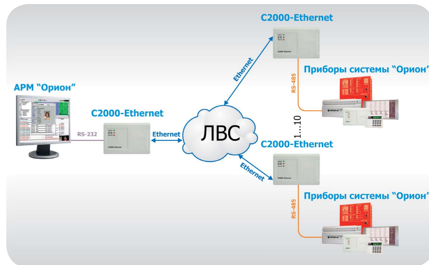
Рисунок 80. Типовая схема работы «С2000-Ethernet» по протоколу «Орион»
