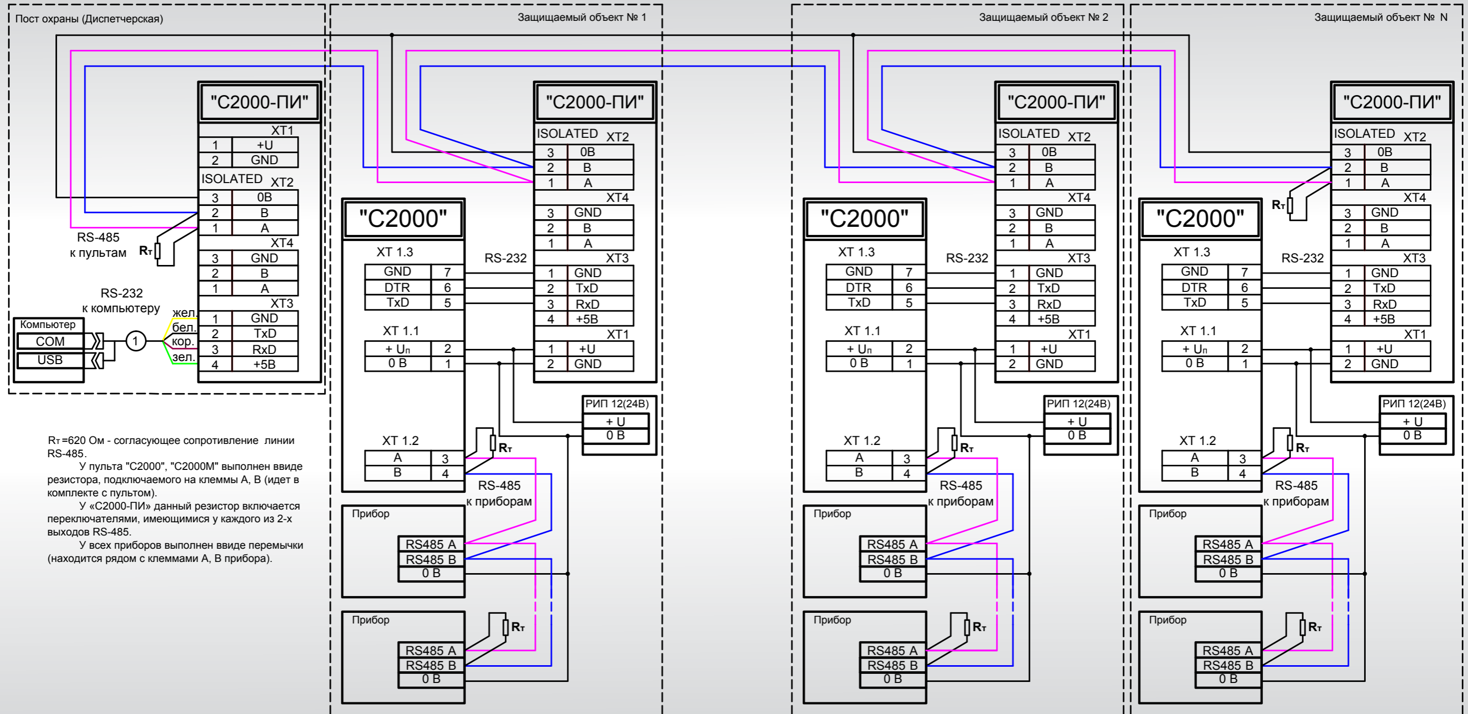
Рисунок 60. Схема подключения нескольких пультов к
