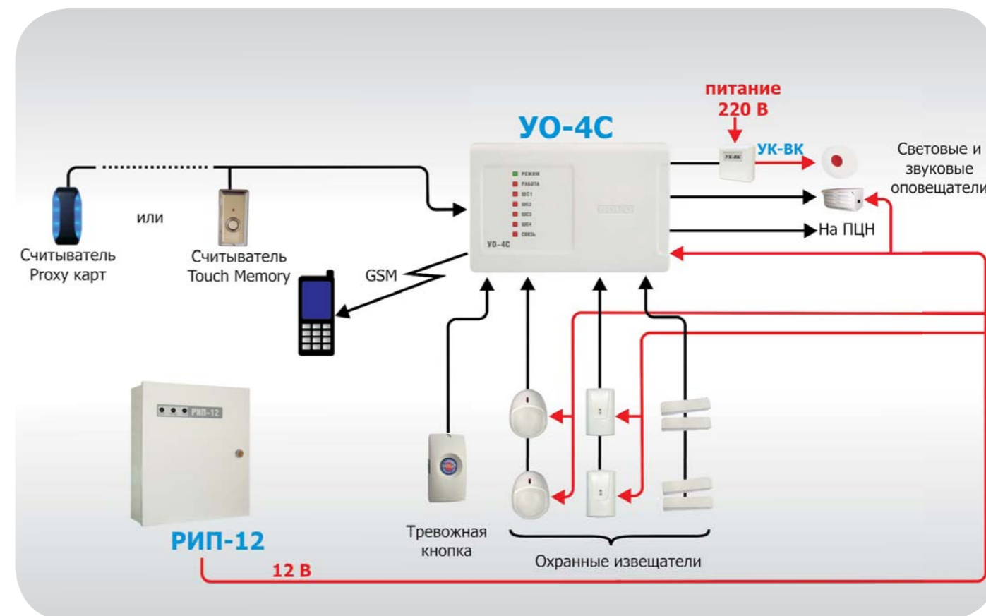
Рисунок 31. Автономное использование «УО-4С»
