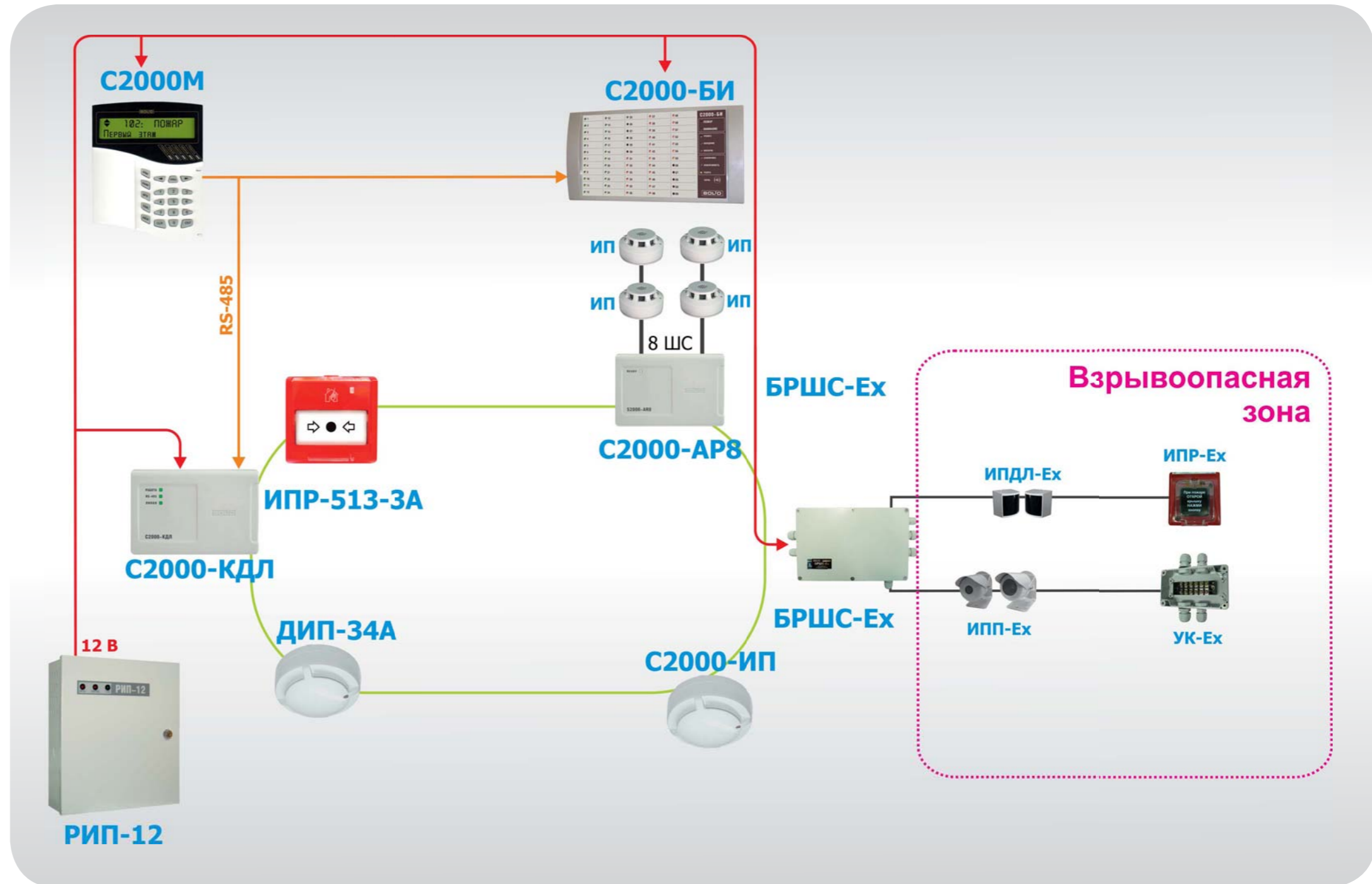
Рисунок 10. Взрывозащищённая система на базе адресно-аналоговой ПС
