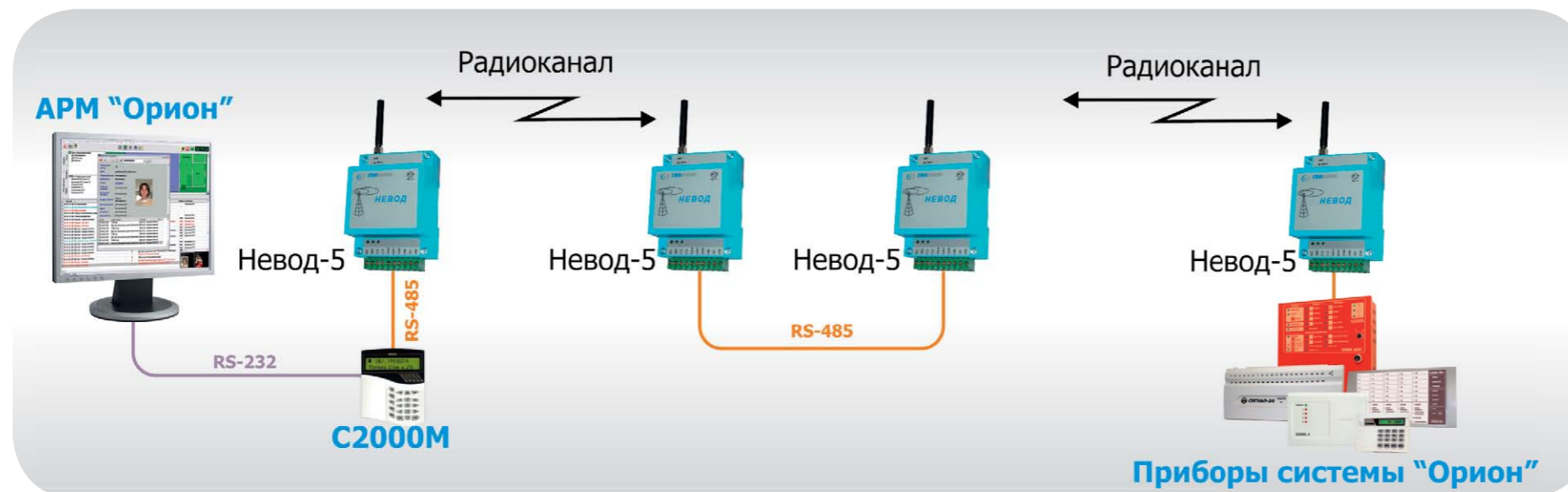
Рисунок 78. Структурная схема использования «Невод-5» с АРМ «Орион» и «С2000М», соединение «точка-точка» с ретрансляцией
