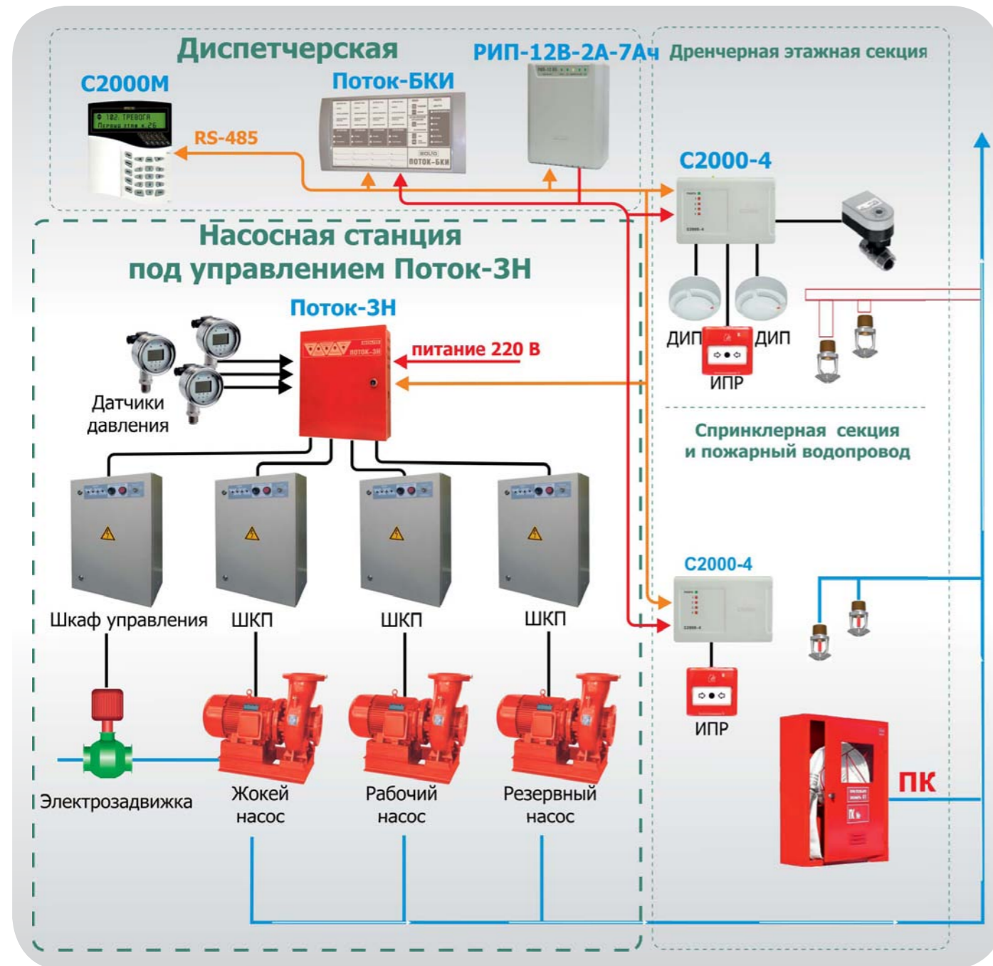
Рисунок 24. Централизованная система водяного пожаротушения
