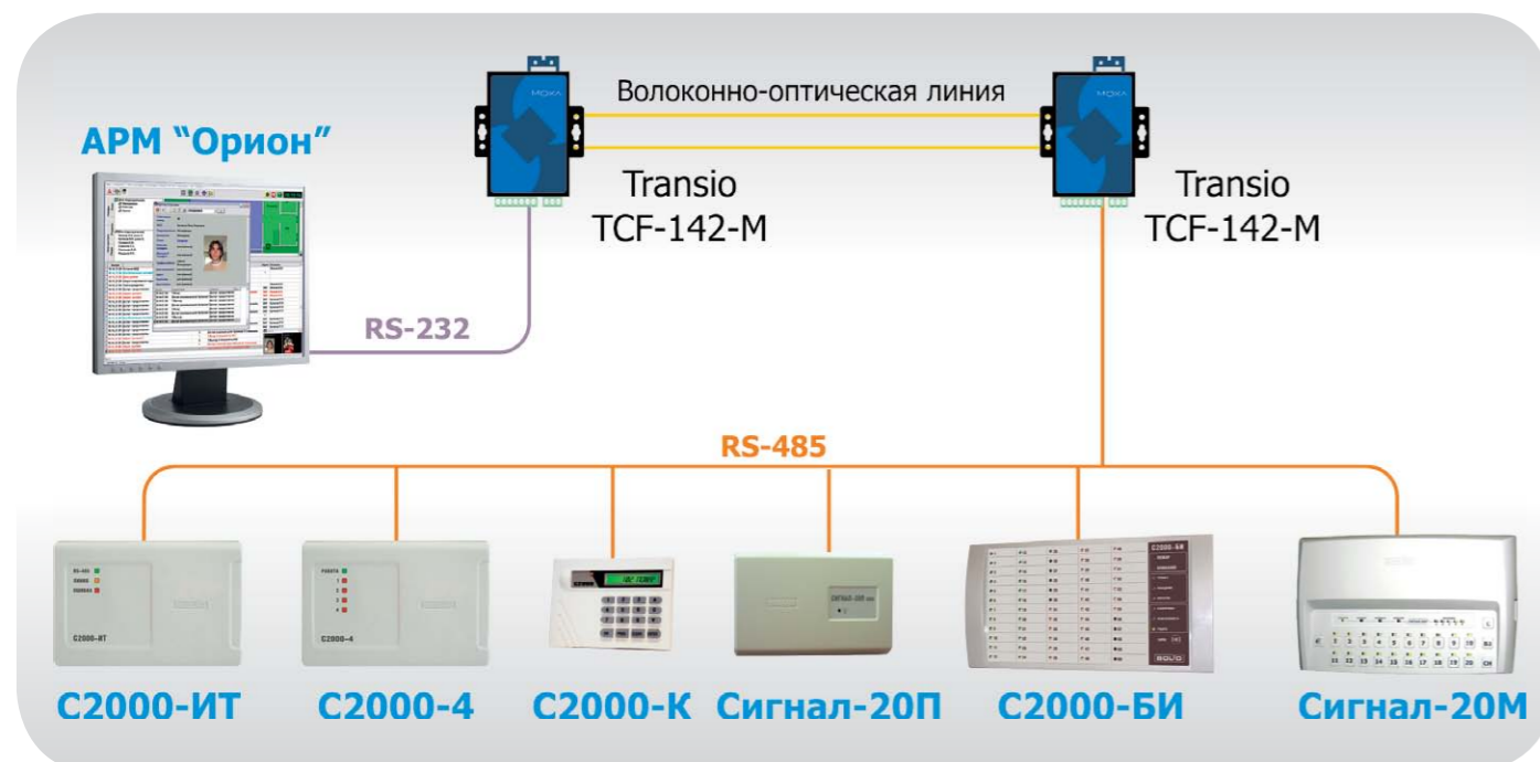
Рисунок 79. Типовая схема работы Transio TCF-142-M по протоколу «Орион»
