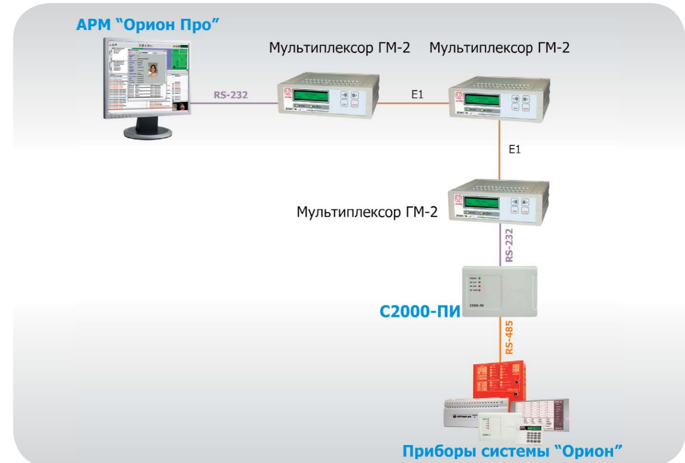
Рисунок 67. Структурная схема использования мультиплексора «ГМ-2» с АРМ «Орион»/«Орион Про» с подключением промежуточного мультиплексора (ремultipлексирование)
