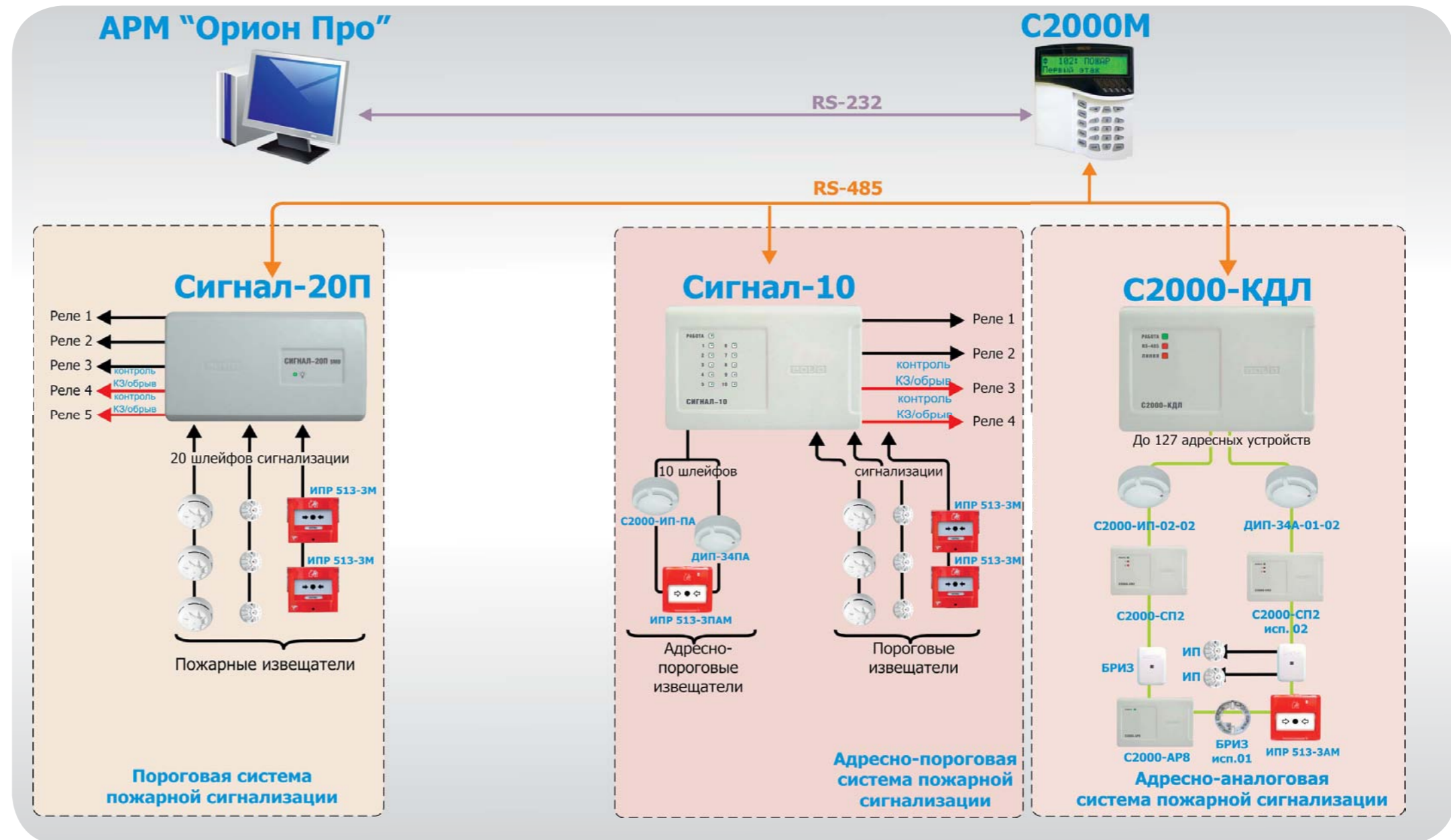
Рисунок 3. Типы систем пожарной сигнализации
