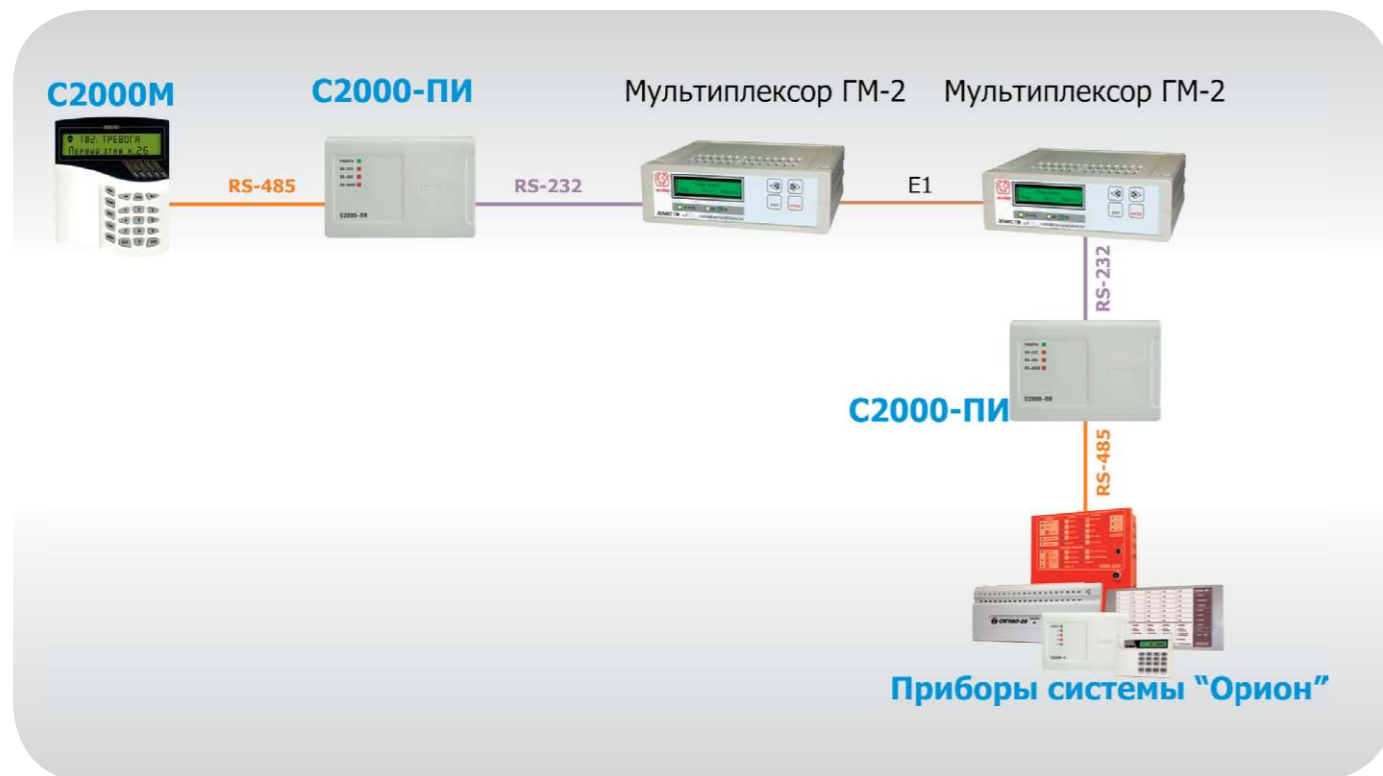
Рисунок 68. Структурная схема использования мультиплексора «ГМ-2» с пультом «С2000М»
