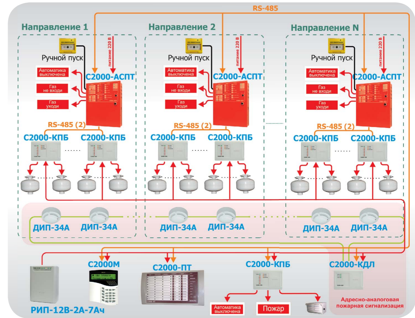
Рисунок 25. Система тушения с использованием адресно-аналоговой пожарной сигнализации
