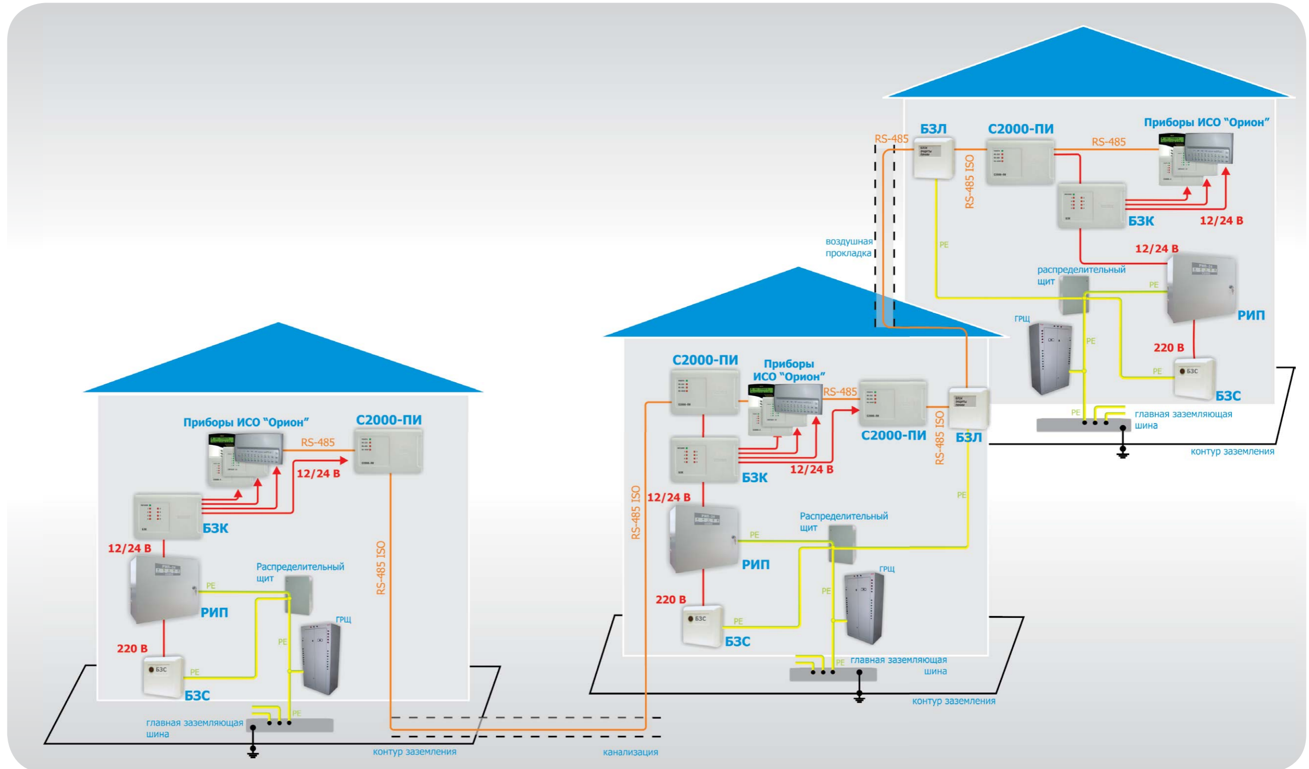
Рисунок 81. Схема подключения приборов с защитой интерфейса RS-485 от перенапряжений
