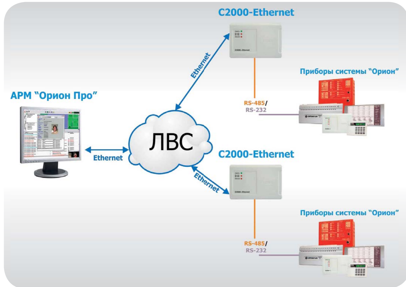
Рисунок 85. Структурная схема использования «С2000-Ethernet» с АРМ «Орион Про» при прямой передаче по ЛВС
