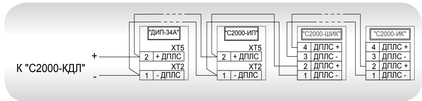
Рисунок 82. Схема подключения адресных извещателей в ДПЛС с топологией построения «шина»
