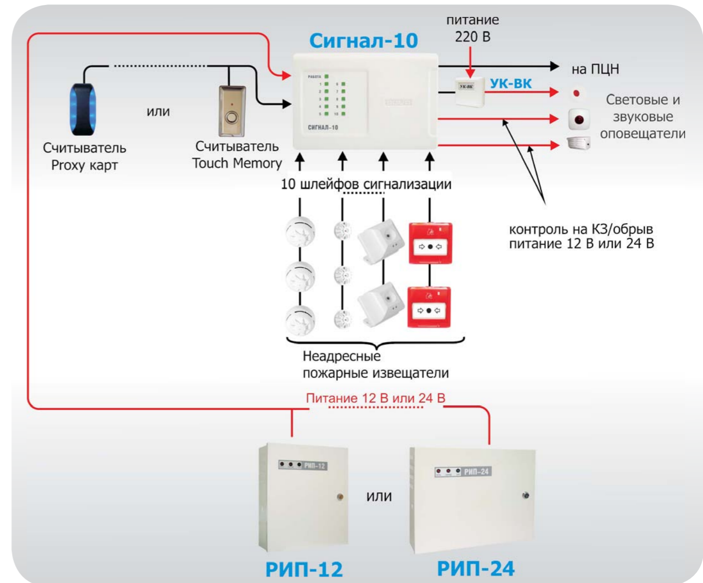
Рисунок 5. Использование прибора «Сигнал-10» в автономном режиме
