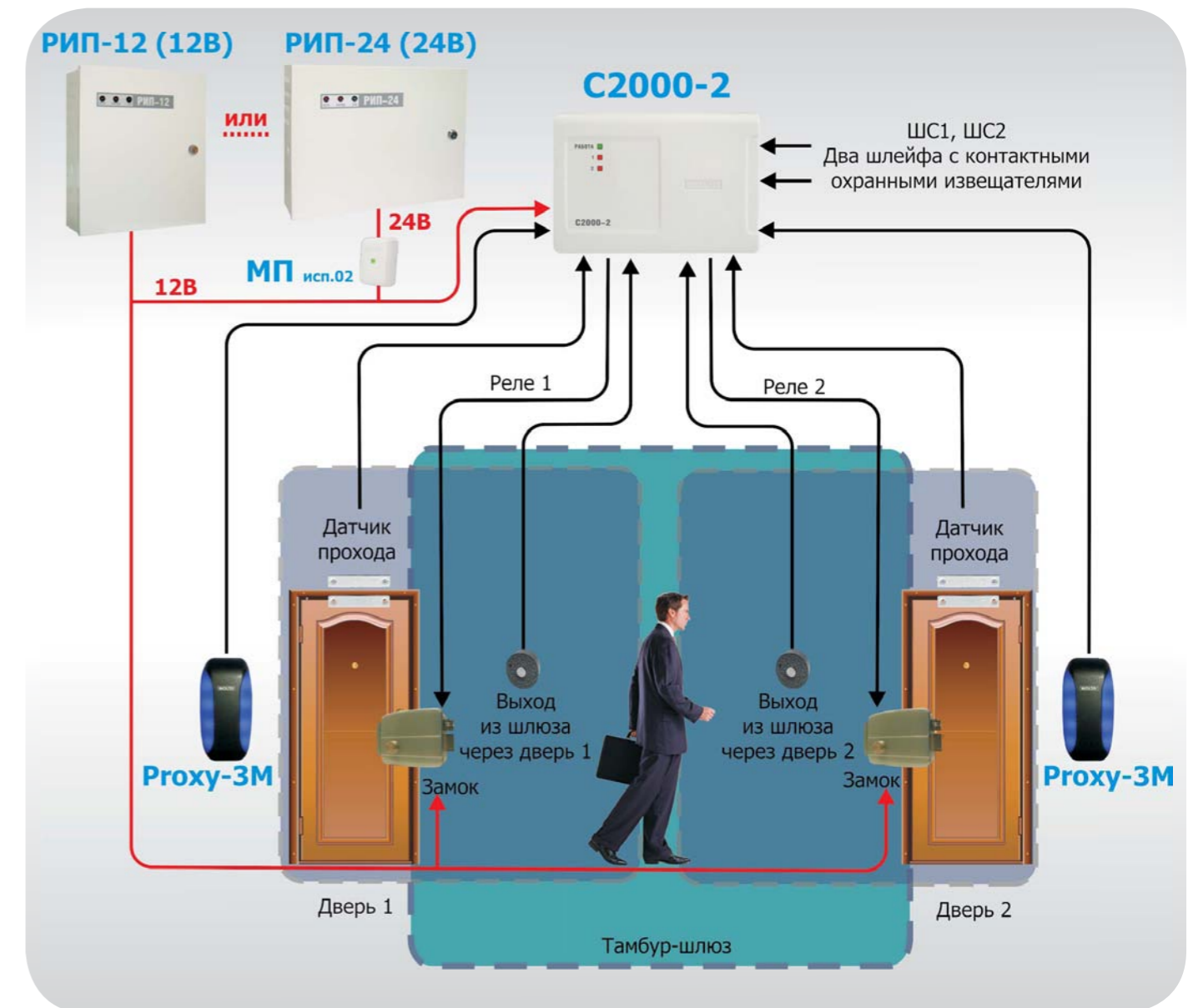
Рисунок 40. Режим работы «Шлюз»
