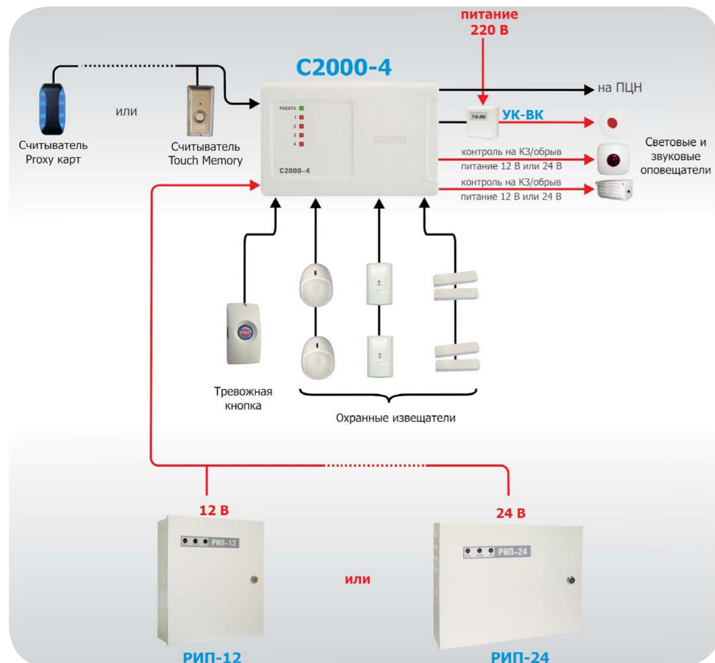
Рисунок 28. Автономное использование прибора «С2000-4»
