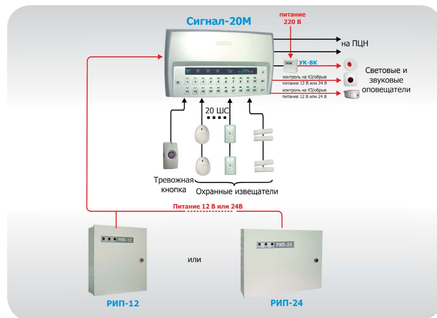
Рисунок 30. Автономное использование прибора «Сигнал-20М»
