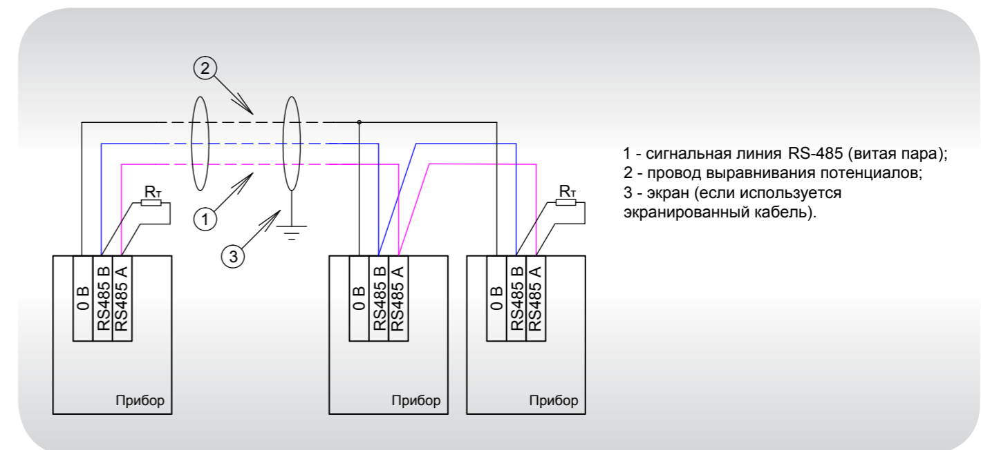
Рисунок 69. Схема подключения приборов к магистральному интерфейсу RS-485
