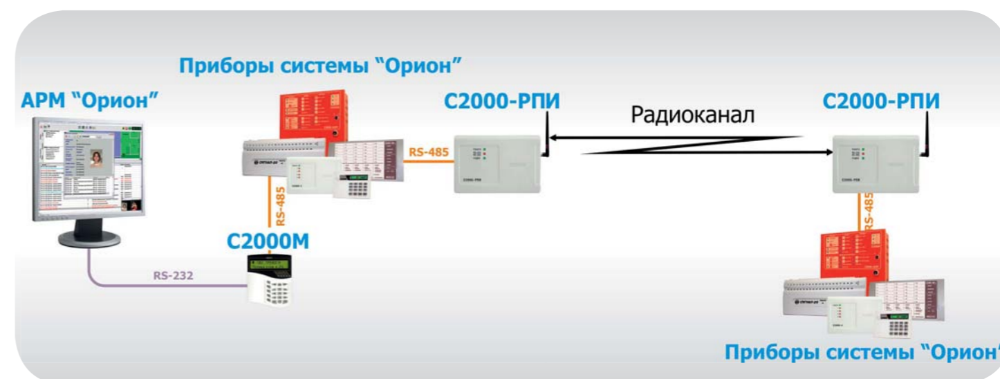
Рисунок 74. Структурная схема использования «С2000-РПИ» с АРМ «Орион» и «С2000М», соединение «точка-точка»
