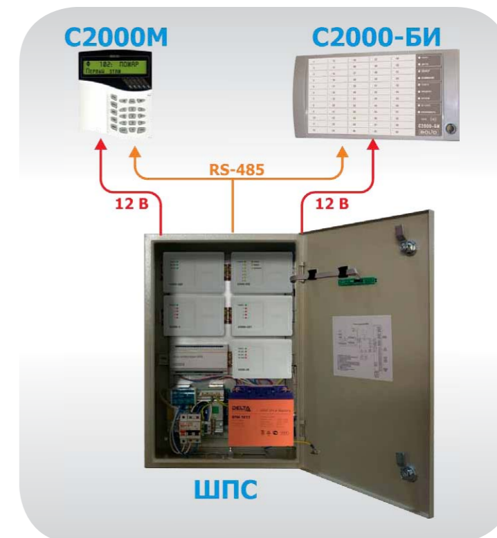
Рисунок 12. Шкаф пожарной сигнализации со встроенным РИП
