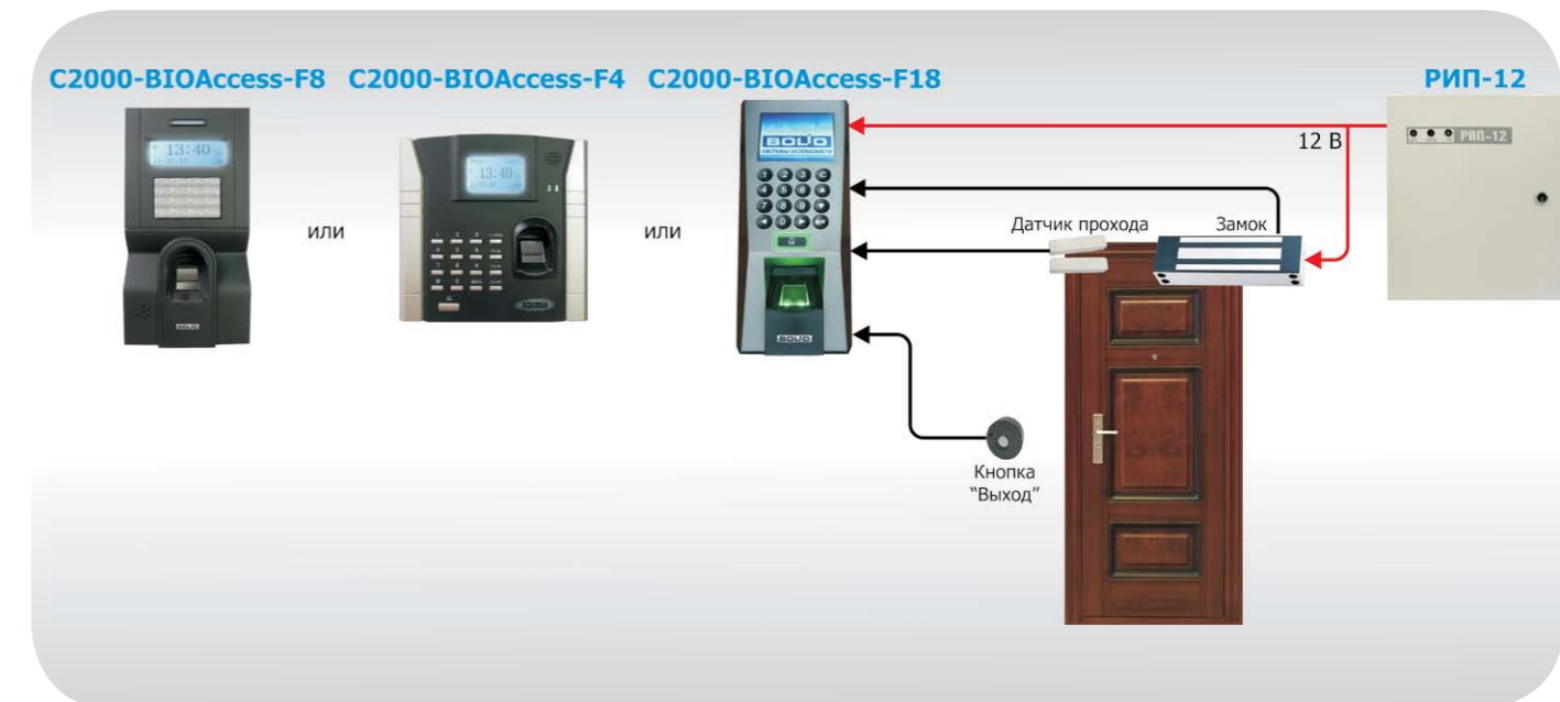
Рисунок 42. «С2000-BIOAccess-F4», «С2000-BIOAccess-F8», «С2000-BIOAccess-F18»
