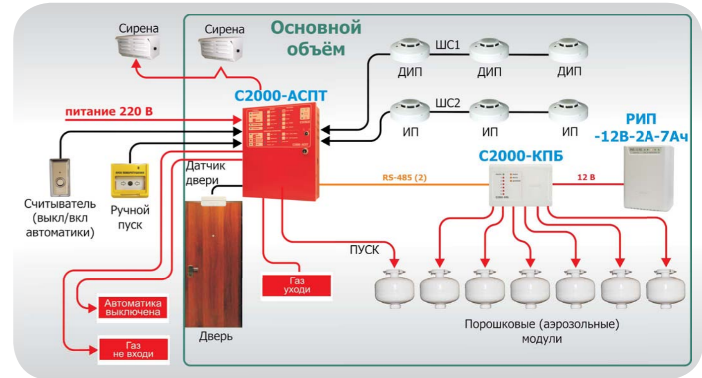
Рисунок 20. Автономная установка порошкового пожаротушения
