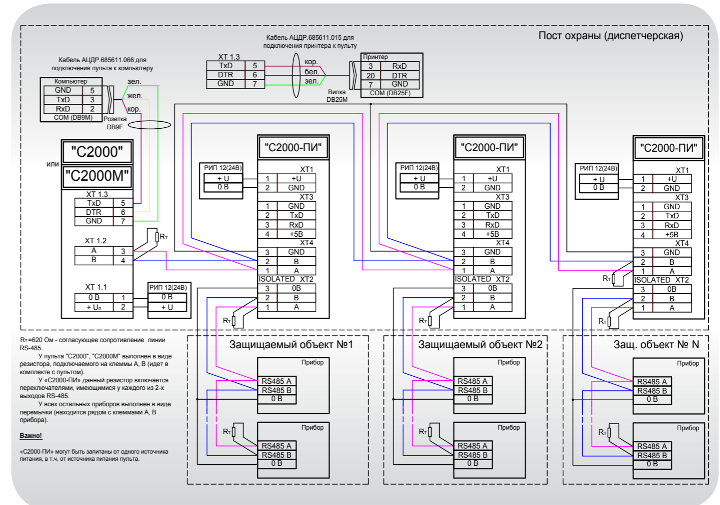
Рисунок 71. Построение сети RS-485 с топологией «звезда» при помощи повторителей
