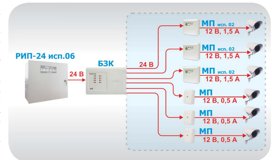
Рисунок 50. Организация электропитания системы видеонаблюдения
