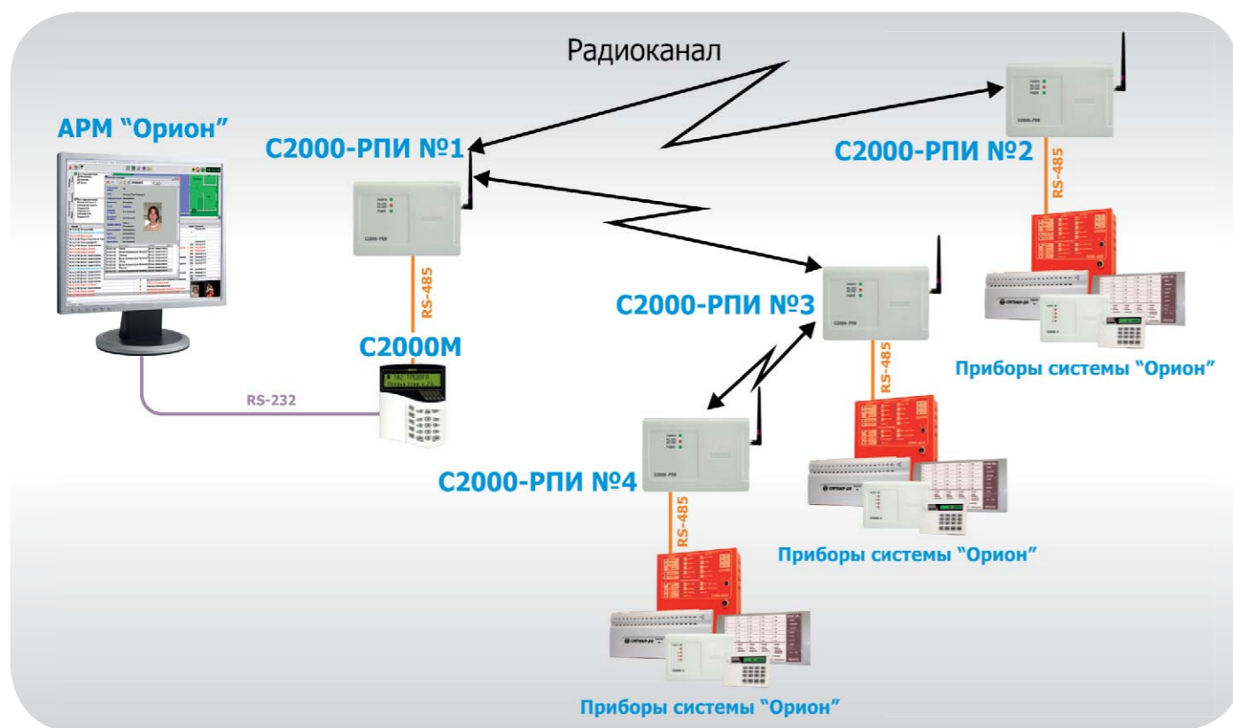
Рисунок 76. Структурная схема использования «С2000-РПИ» с АРМ «Орион» и «С2000М», соединение «точка-многоточие» с ретрансляцией
