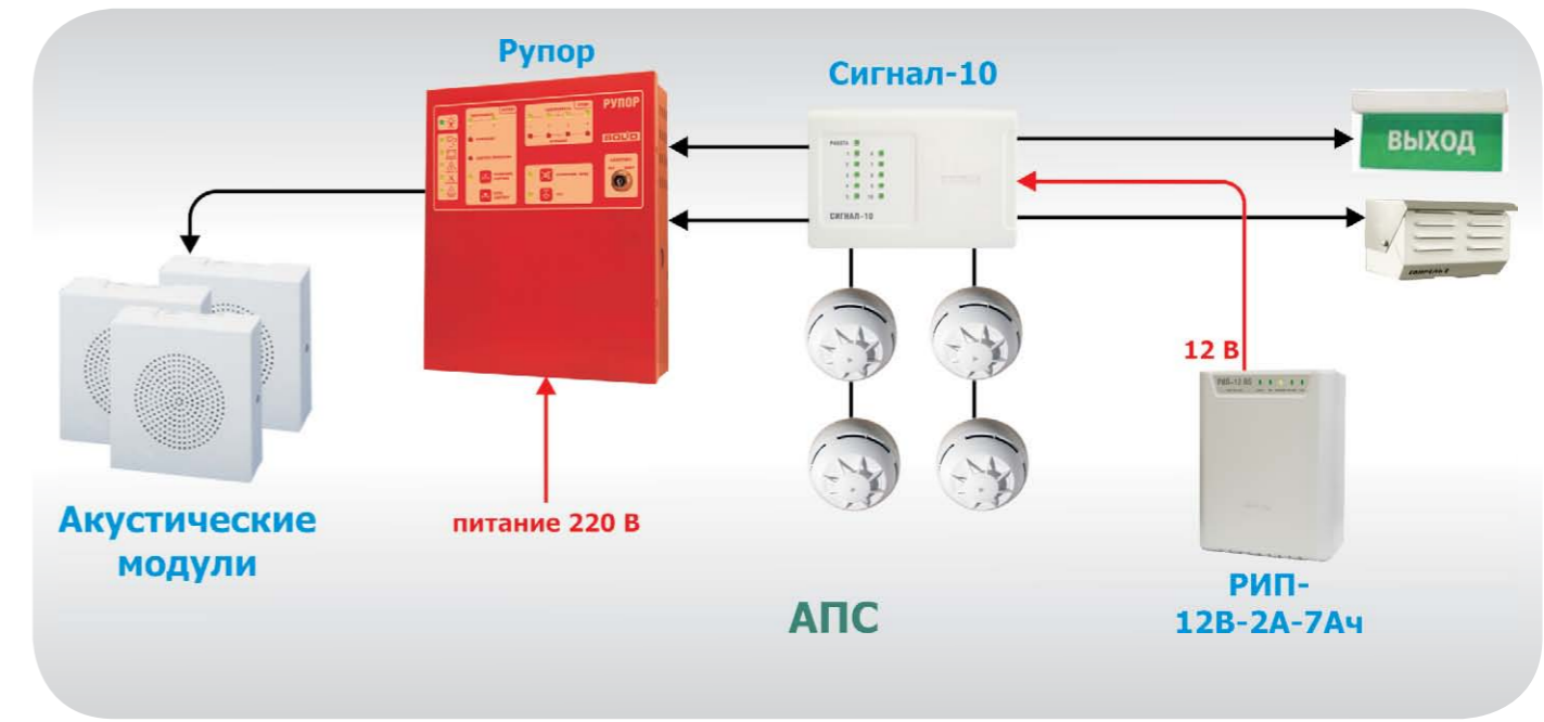
Рисунок 15. Пример СОУЭ 3-го типа с одной зоной оповещения
