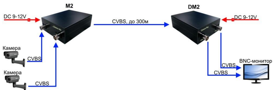
Рис. 7 Схема подключения модулятора M2 и демодулятора DM2. Технические характеристики
